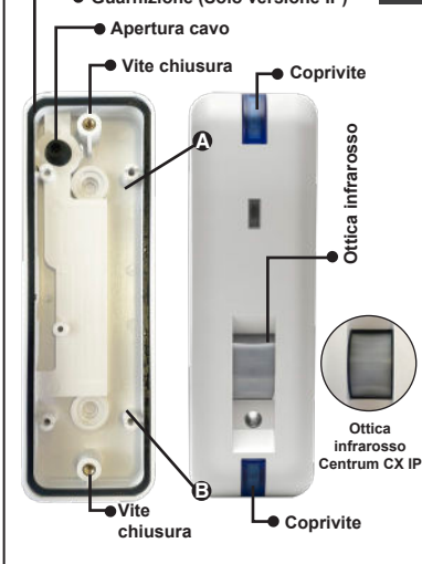
Guarnizione (Solo versione IP) Fig.4
